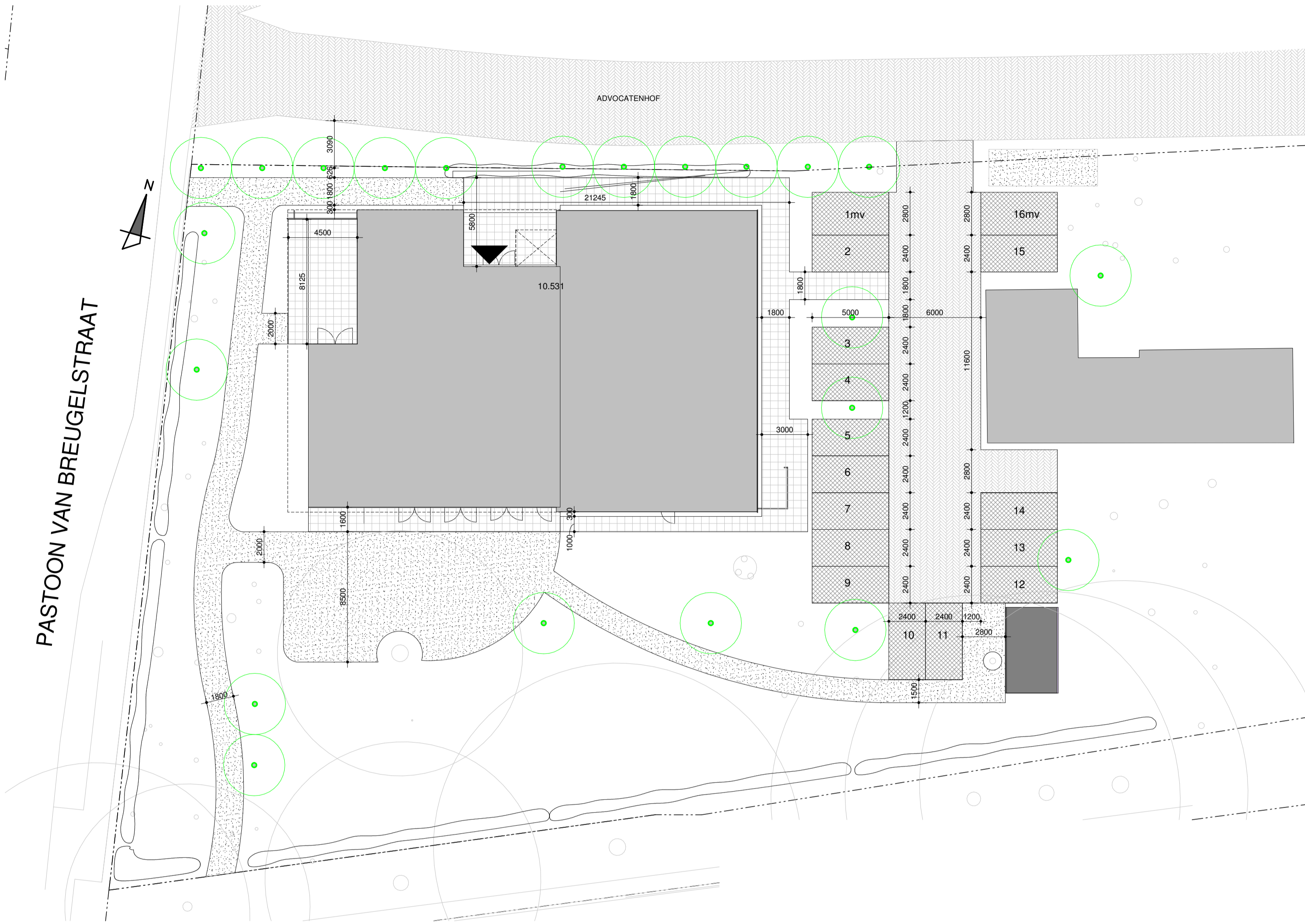
situatie
